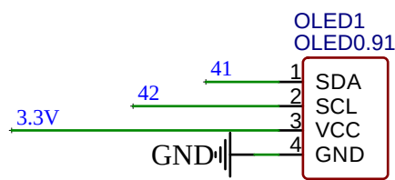
屏幕4P排母
