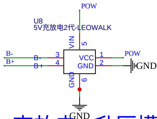
充放电+升压模块
