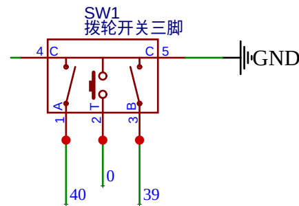
拨轮开关三脚（音量加减和打断对话）
