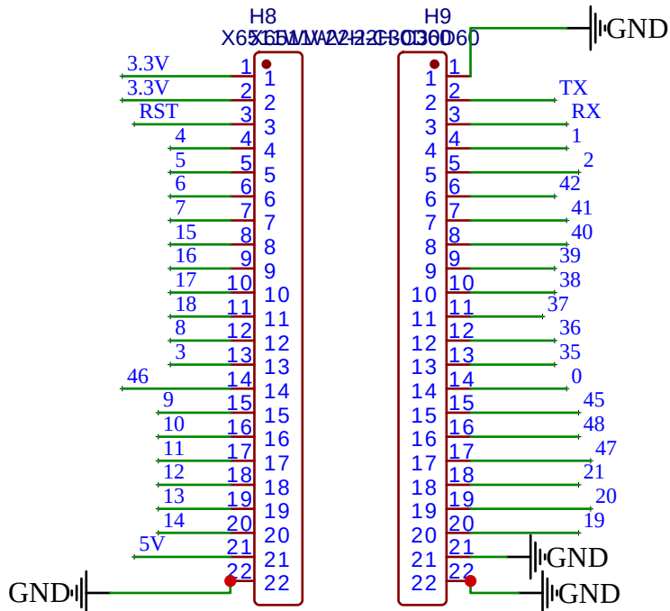
S3拓展引脚，可省略
