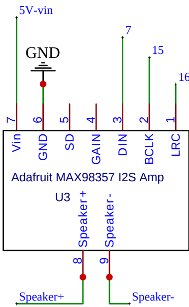
Adafruit MAX98357
