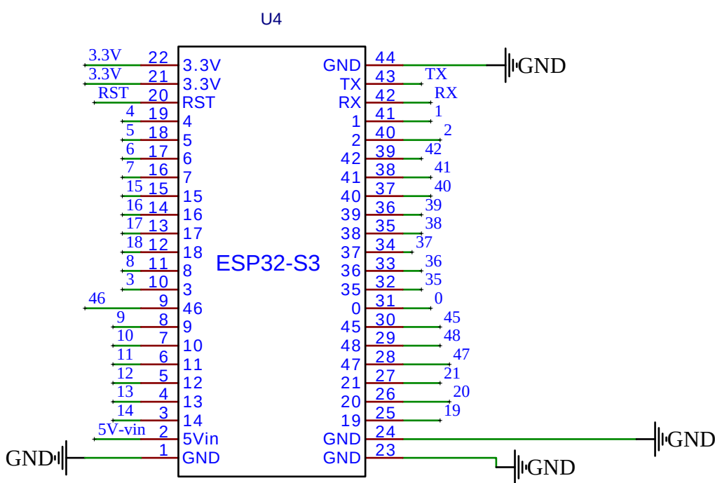
ESP32-S3开发板
