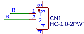
电池拔插式母座
