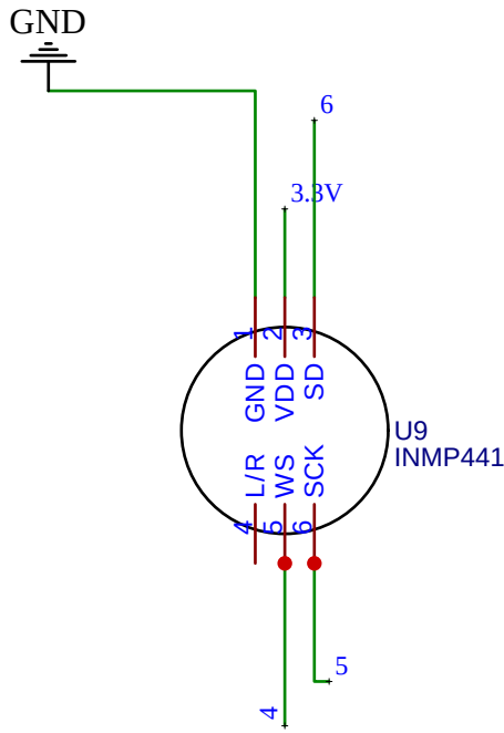
INMP441麦克风
